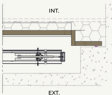
Coupe horizontale
