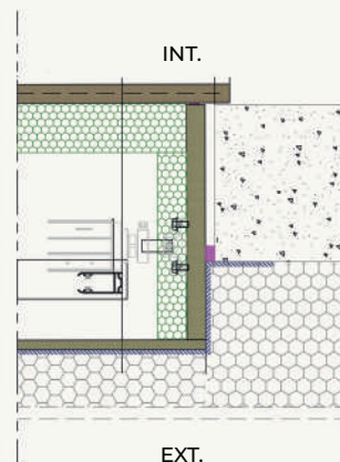
Coupe Horizontale
