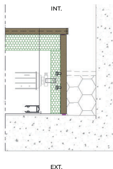
Coupe horizontale
