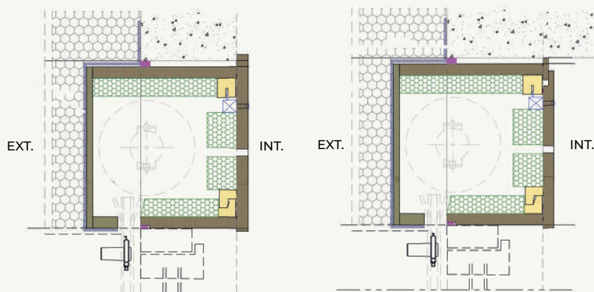
Coupes verticales au nu extérieur
