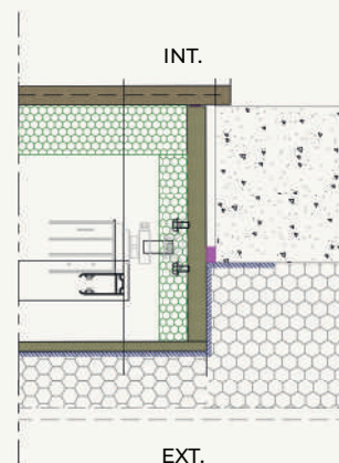
Coupe Horizontale
