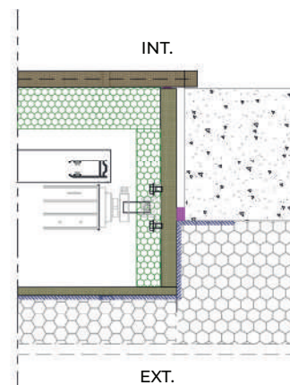
Coupe horizontale
