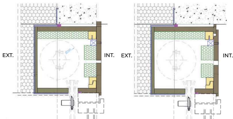
Coupe verticale au nu intérieur
