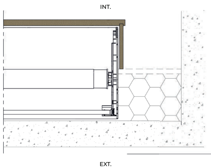
Coupe horizontale
