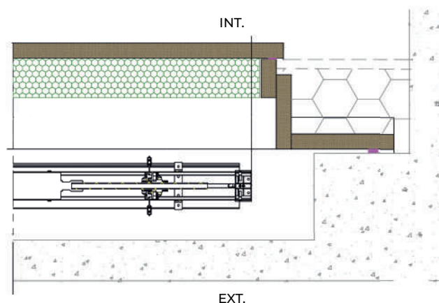
Coupe horizontale
