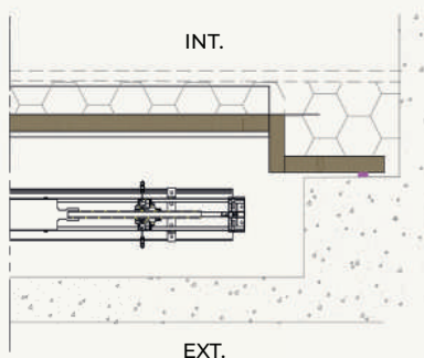
Coupe horizontale
