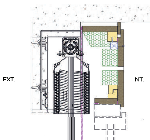
Coupe verticale
