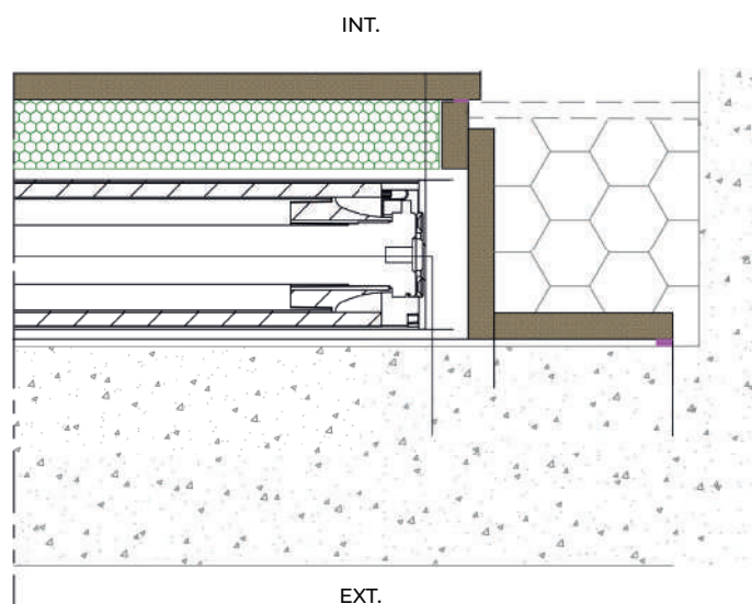
Coupe horizontale
