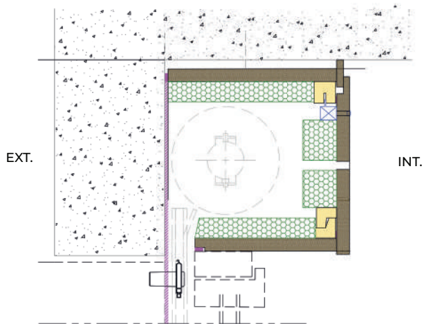
Coupe verticale
