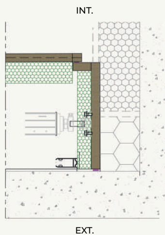
Cloison en butée sur coffre
